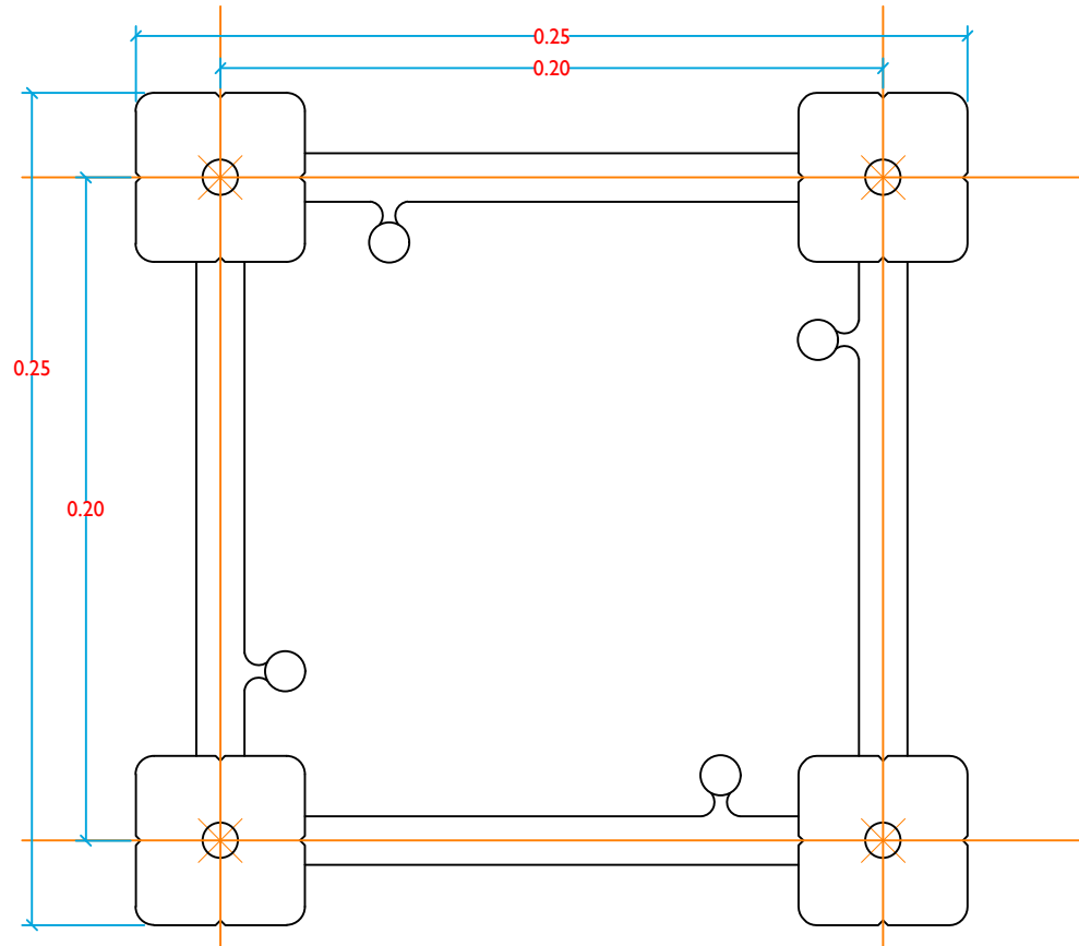
CONDUCTO4 - PLANTA SIN ESCALA
