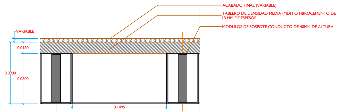
CONDUCTO4 - ELEVACIÓN SIN ESCALA
