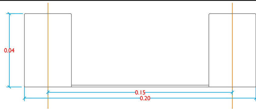
CONDUCTO4 - ELEVACIÓN SIN ESCALA
