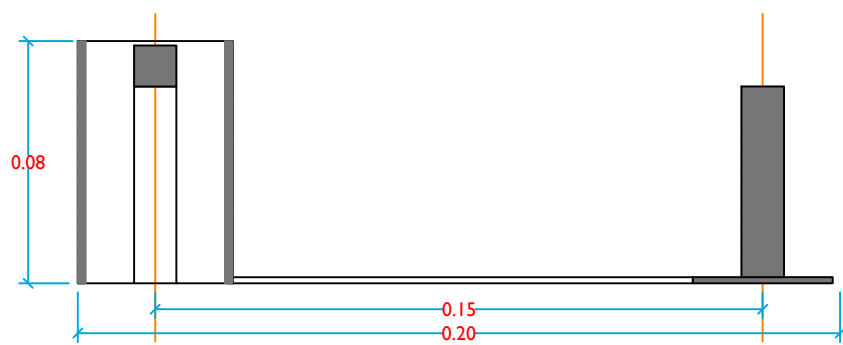
CONDUCTO4 - ELEVACIÓN SIN ESCALA
